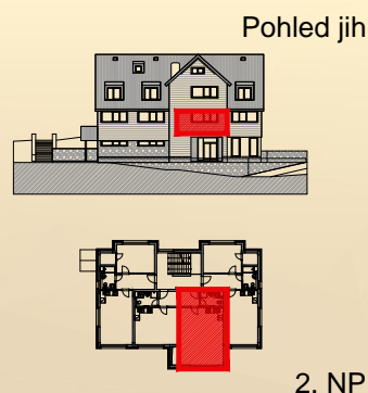
2. NP
